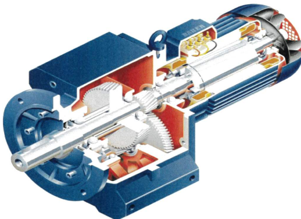
Слика 1. Bauer Geared Motors GmbH мотор-редуктор
